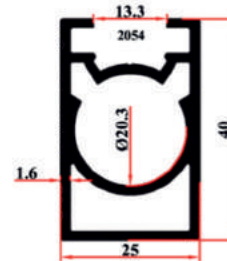
KRM 9135 40x25 Tek Kanallı 0,774 Kg/Mt
