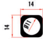
KRM 9132 14x14 Kare Profil 0,255 Kg/Mt
