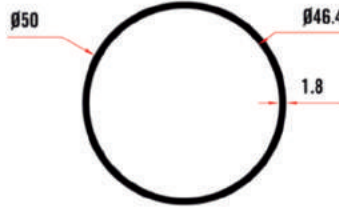
KRM 9102 50x1,8 mm Profil 0,750 Kg/Mt
