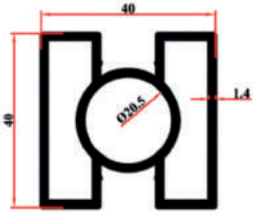
KRM 9125 40x40 Çift Kanallı 0,890 Kg/Mt
