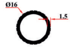
KRM 9120 16x1,5 mm Tırtırlı Boru 0,175 Kg/Mt
