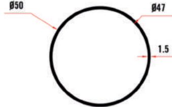
KRM 9103 50x1,5 mm Profil 0,625 Kg/Mt
