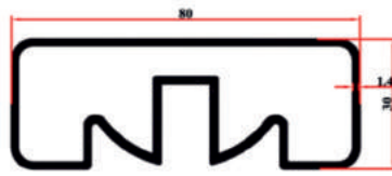
KRM 9122 80x30 Ortadan Kanallı 1,147 Kg/Mt
