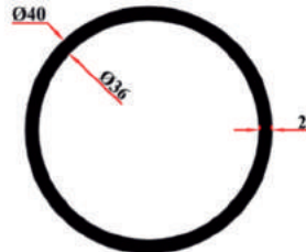
KRM 9106 40x2 mm Boru 0,644 Kg/Mt
