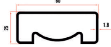
KRM 9123 60x25 Kutu Profil 0,845 Kg/Mt
