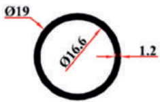
KRM 9117 19x1,2 mm Boru 0,181 Kg/Mt
