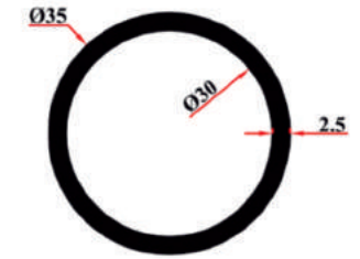
KRM 9112 35x2,5 mm Boru 0,691 Kg/Mt
