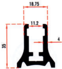
KRM 9133 50'lik Alt Mini Gemici Profil 0,955 Kg/Mt
