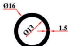
KRM 9118 16x1,5 mm Boru 0,184 Kg/Mt
