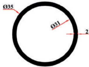
KRM 9113 35x2 mm Boru 0,561 Kg/Mt
