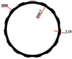
KRM 9105 50'lik Tırtırlı Boru 0,730 Kg/Mt
