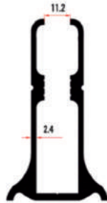
KRM 9134 50'lik Alt Kızak Profil 1,755 Kg/Mt
