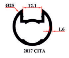
KRM 9116 25'lik Kanallı Boru 0,472 Kg/Mt
