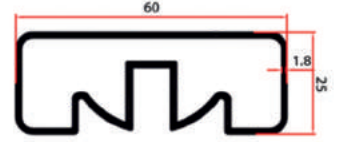
KRM 9124 60x25 Ortadan Kanallı 0,865 Kg/Mt
